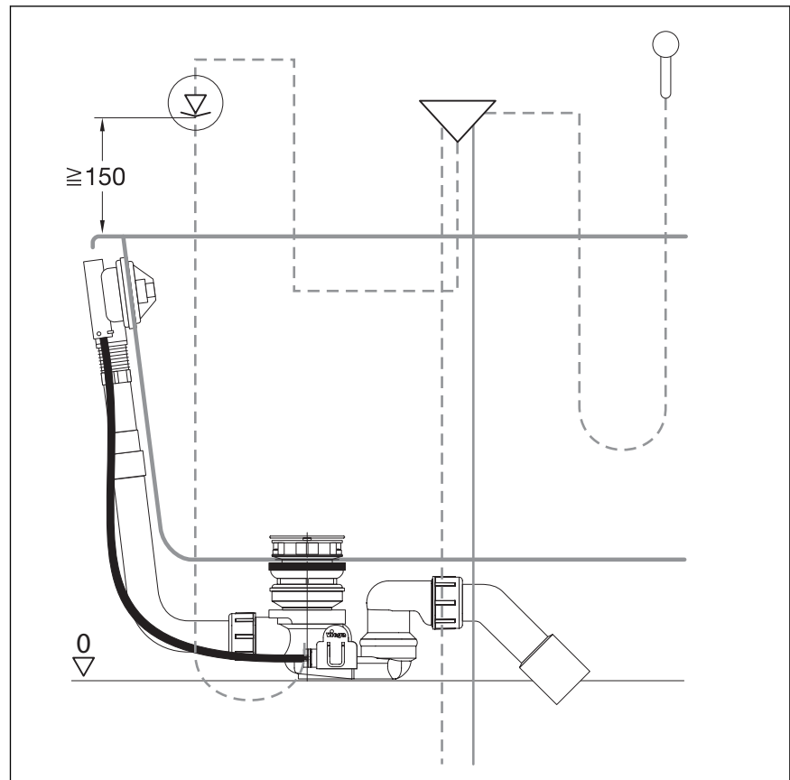
Abb. 4: Mindesteinbauhöhe 150 mm
