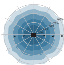
Avec installation au plafond (Unité : m) Hauteur d'installation suggérée : 2,5 - 6 m
