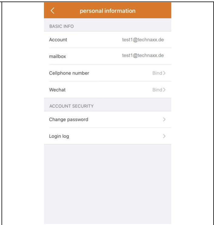
Benutzerinformationen (Konto)
