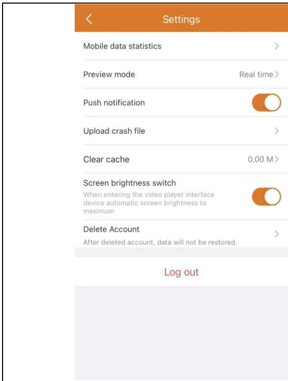
Einstellungen (App)
