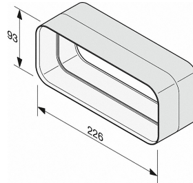
DFK-V, Flachkanal-Verbinder, Skizze
